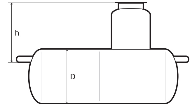
Горизонтальная ёмкость:
